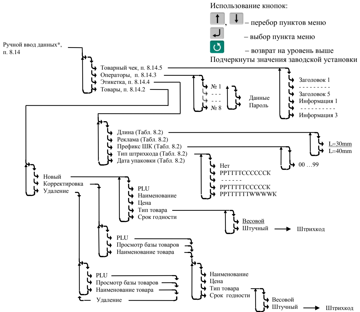
Рис. 8.2 – Схема заполнения справочников с клавиатуры терминала
