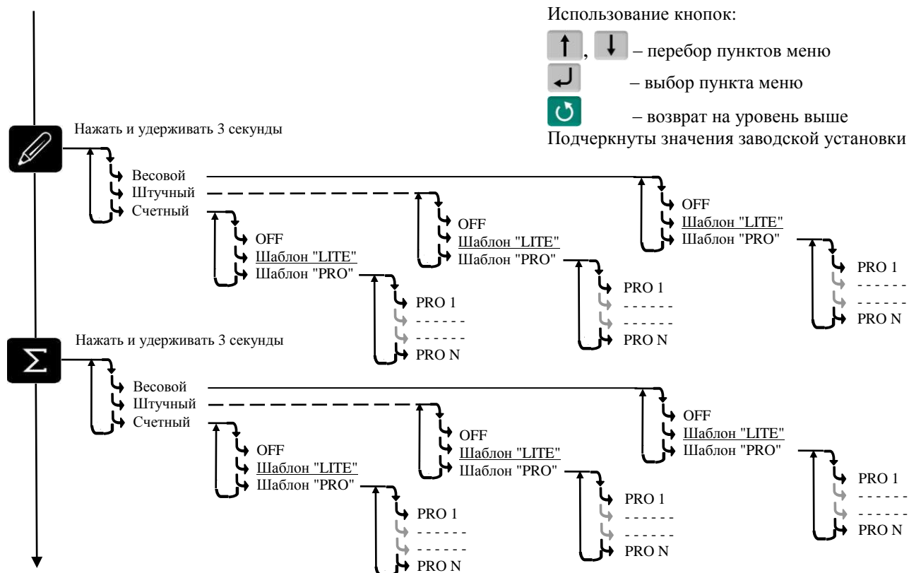
Рис. 4.2 – Схема установки шаблонов печати
